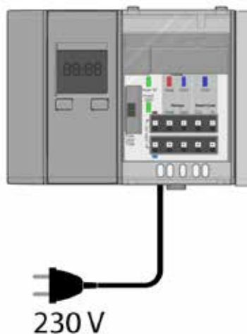
Afbeelding 3: Basismodule-regelaar met timer-unit
