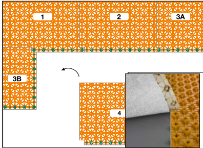
8 Die Verlegerichtung ist durch die, in der Darstellung grün gekennzeichneten, verjüngten Verbindungs­noppen vorgegeben. Abschnitte \geq 30 cm können am Beginn der nächsten Reihe eingespart werden. Das Einrasten der Noppenplatten erfolgt auf den verjüngten Verbindungs­noppen. Um Schallbrücken zu vermeiden, müssen die Noppen der EN 18 FTS im Randbereich zur Wand entfernt werden.
