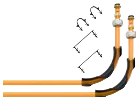
Onderdelen van aansluitset voor verwarmingsbuis Ø 16 mm
